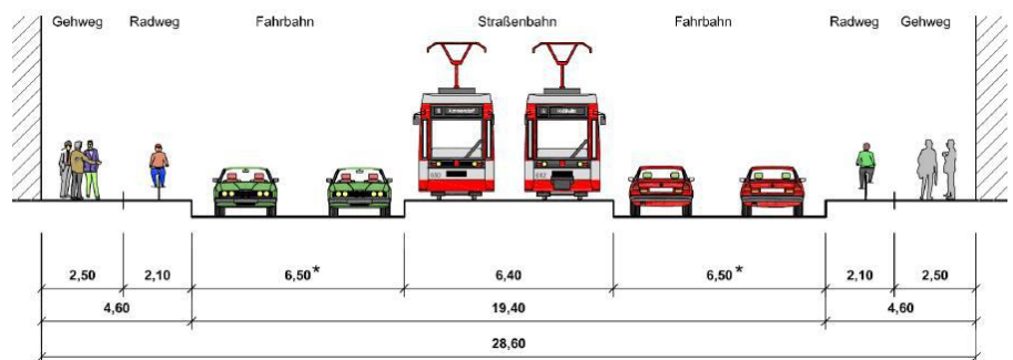
Bild 1: Varianten I EÜ Merseburger Straße km 3,91 (6343) mögliche Ansicht
